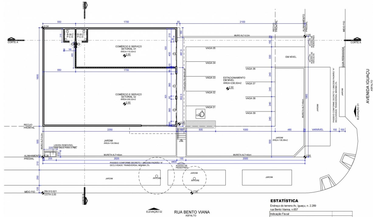
PLANTA DO PAVIMENTO TÉRREO ESCALA 1:100
